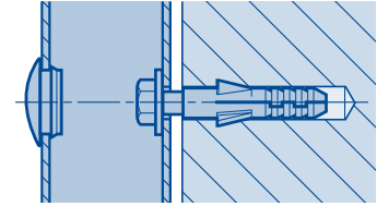
Verschraubung durch die Zarge
